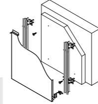
KASET TİPİ V1 CASSETTE TYPE V1
