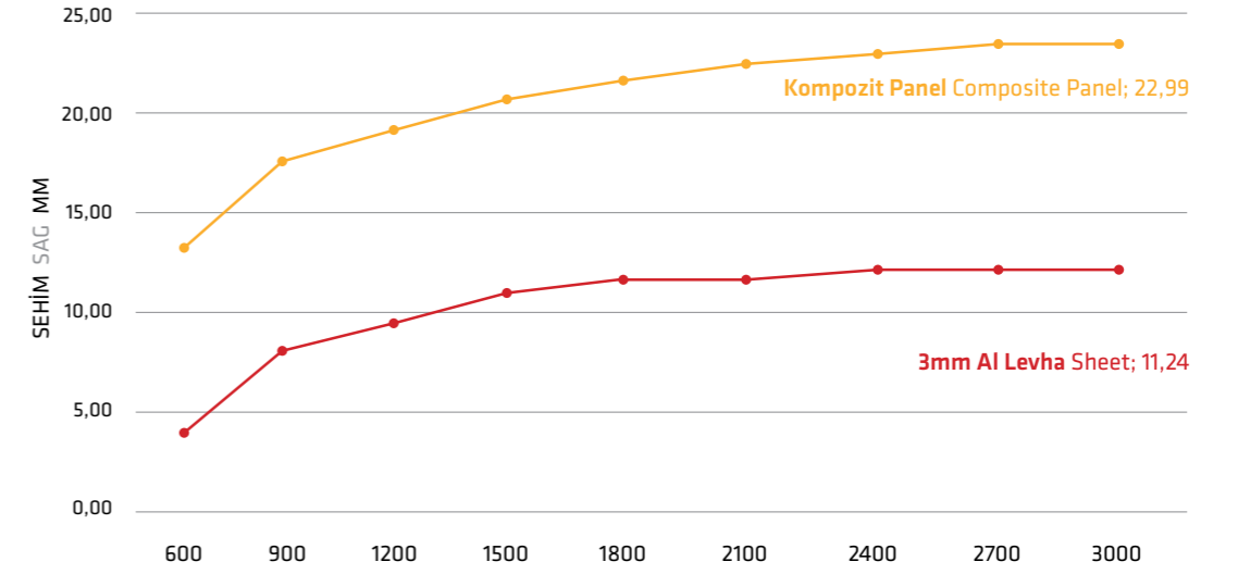
SEHİM SAG
